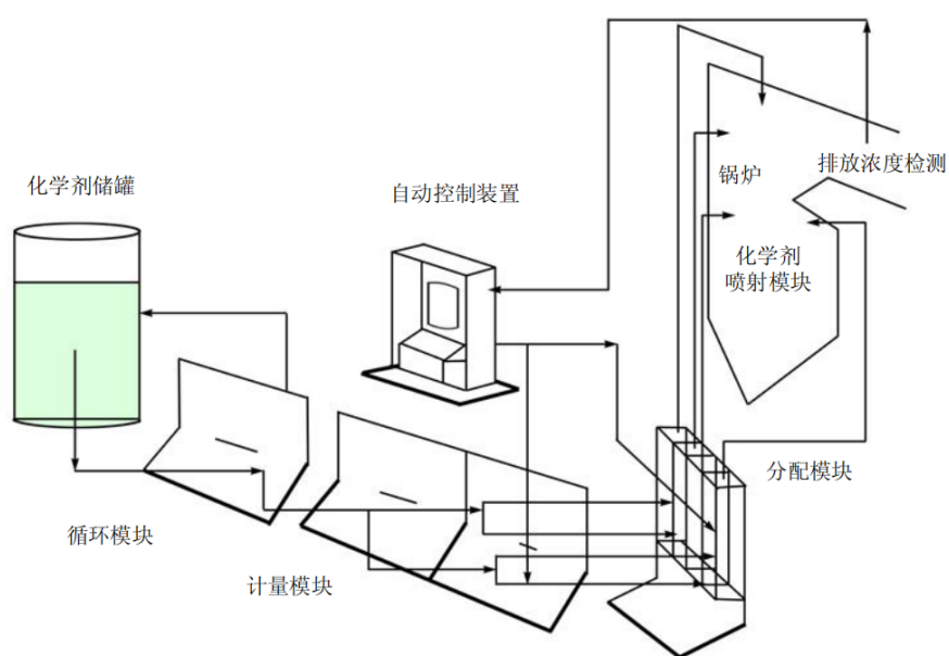
图 B.2 模块的供给系统
