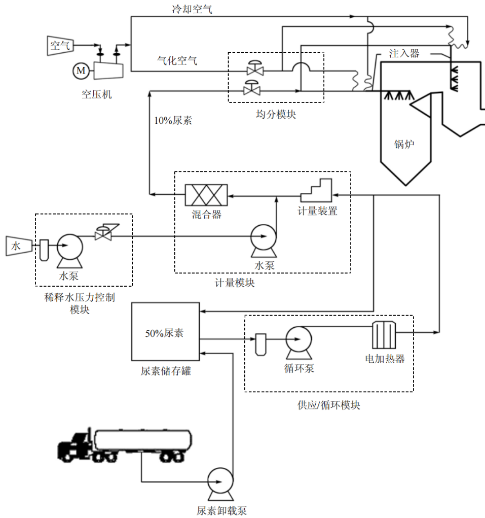
图 B.1 尿素 SNCR 系统工艺
